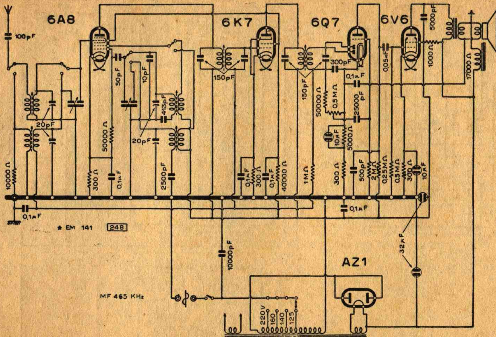
Lo schema elettrico del mod. 514
